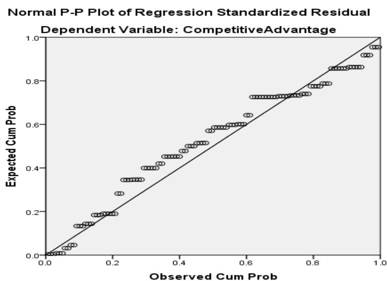
الشكل (4 - 2): اختبار الخطية: العلاقة بين المتغير المستقل والمتغير التابع علاقة خطية
