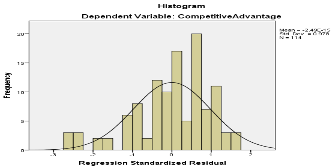
الشكل (4 - 1): التوزيع الطبيعي
