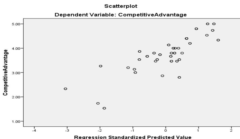
الشكل (3-4): اختبار العلاقة الخطية
