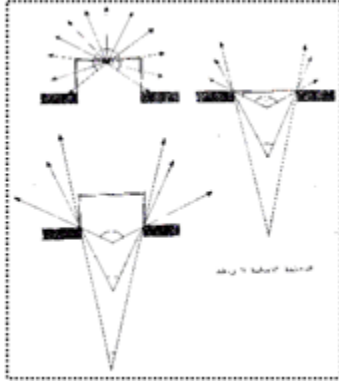
شكل (٣-٦): نوافذ وقبة قاعة الأختين (الاتصال بين الأرض والسماء) شكل (٣-٧): خطوط الرؤية (معالجة النوافذ في العمارة الأندلسية). المصدر: تحليل الباحث.
