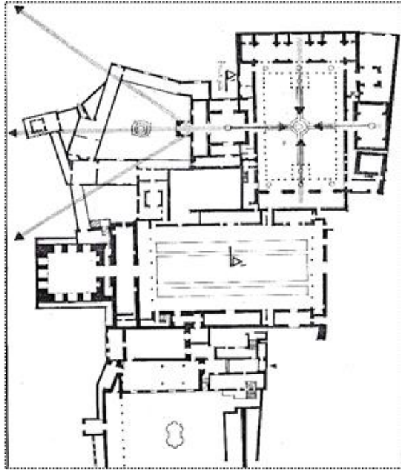
شكل (٣-٣): المحاور القوية من السمات الأساسية لعمارة القصور الأندلسية حيث تتفاعل مع التكوينات الفراغية لتؤكد المعاني الكائنة وراء تلك التكوينات في إطار من السيمتزية الغالبة المصدر: تحليل الباحث.
