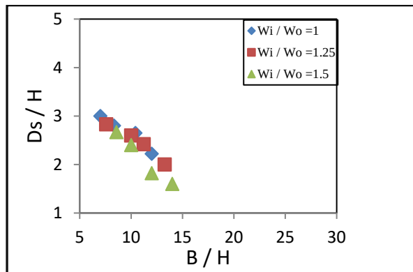
شكل (16) علاقة نسبة عمق النحر D_s/H والطول الجانبي للهدار B/H الى ارتفاع الماء فوق الهدار عند 90 سم L_b و 25 سم p
