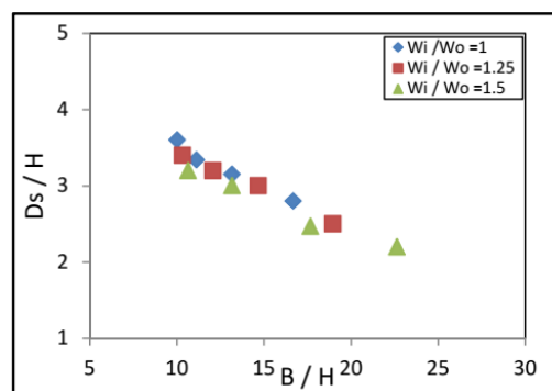
شكل (17) علاقة نسبة عمق النحر D_s/H والطول الجانبي للهدار B/H الى ارتفاع الماء فوق الهدار عند L_b = 90 سم و p=30 سم
