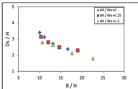
شكل (20) علاقة نسبة عمق النحر D_s/H والطول الجانبي للهدار B/H الى ارتفاع الماء فوق الهدار عند L_b = 120 سم و p=30 سم
