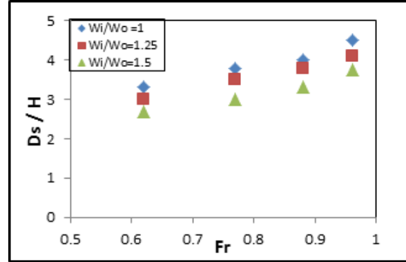
شكل (15) علاقة نسبة عمق النحر الى ارتفاع الماء فوق الهدار D_s/H ورقم فرود للهدار مفتاح البيانو عند P=35 سم و L_b=120 سم
