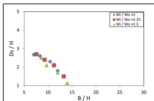
شكل (19) علاقة نسبة عمق النحر D_s/H والطول الجانبي للهدار B/H الى ارتفاع الماء فوق الهدار عند L_b = 120 سم و p=25 سم
