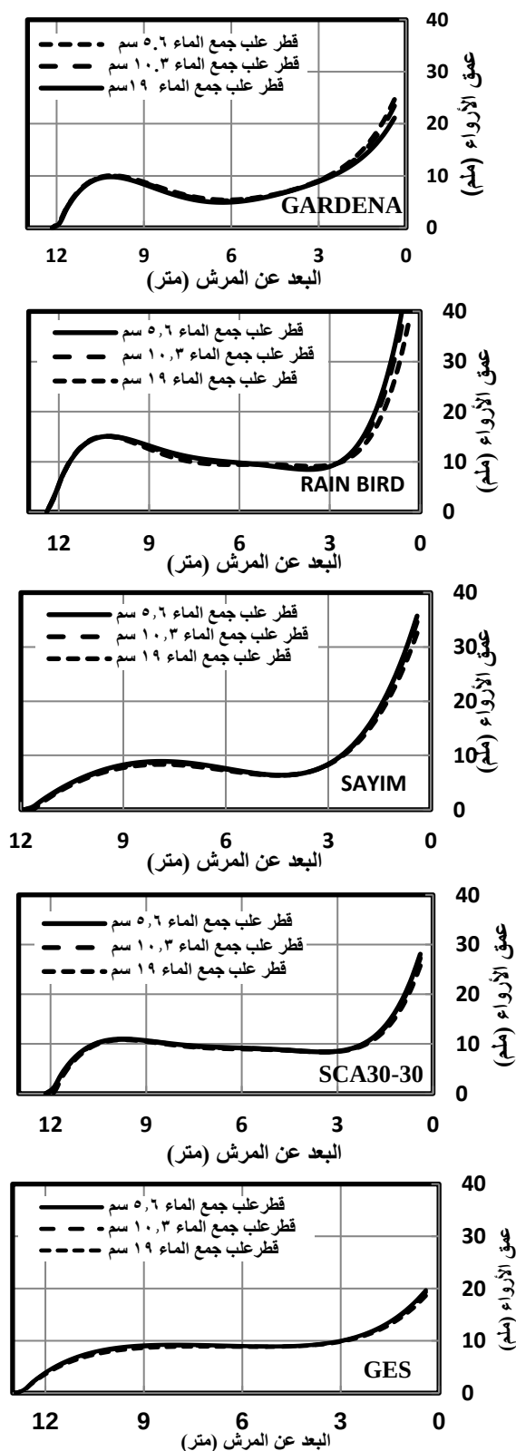
الشكل (9): نمط توزيع الماء على امتداد الشعاع الذي يمثل نصف قطر دائرة الابتلال مركزها المرشدة باستخدام علب جمع الماء بأقطار مختلفة ولعدة رؤوس للمرشات.
