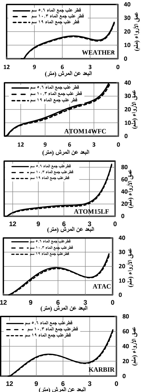
الشكل (10): نمط توزيع الماء على امتداد الشعاع الذي يمثل نصف قطر دائرة الابتلال مركزها المرشحة باستخدام علب جمع الماء بأقطار مختلفة ولعدة رؤوس للمرشحات.
