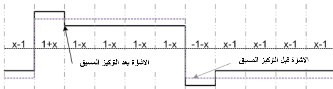
الشكل (3) يوضح شكل الإشارة قبل وبعد عمل التركيز المسبق
