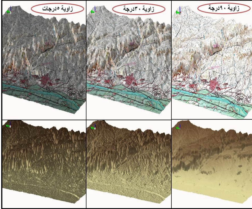
المصدر: من إعداد الباحث اعتماداً على برنامج Arc Sene10.5 شكل ١٥: اختلاف تأثير الإضاءة وفقاً لموضع الشمس الافتراضي لمنطقة الدراسة
