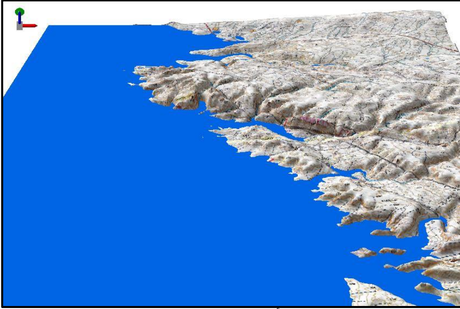
المصدر: من إعداد الباحث اعتماداً على برنامج Arc Sene10.5 شكل ٢٦: نموذج محاكاة ثلاثي الأبعاد لمخاطر السيول والفيضانات على منطقة الدراسة
