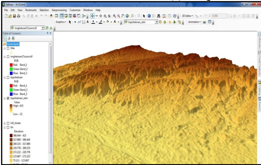
المصدر: من إعداد الباحث اعتماداً على برنامج Arc Sene10.5 شكل ٢: نموذج ثلاثي الأبعاد لنموذج الارتفاع الرقمي لمنطقة الدراسة من واجهة برنامج (Arc scene)
