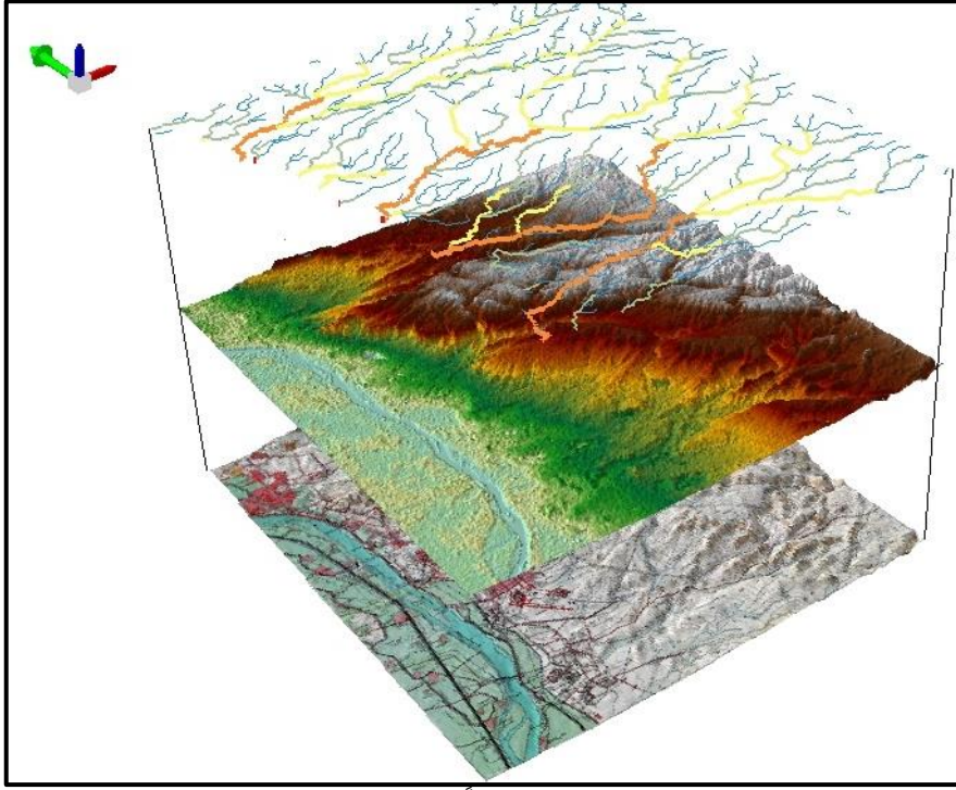
المصدر: من إعداد الباحث اعتماداً على برنامج Arc Sene10.5 شكل ٢٥ : استنباط شبكة الأودية ورتبها من الخريطة الطبوغرافية ونموذج الارتفاع الرقمي
