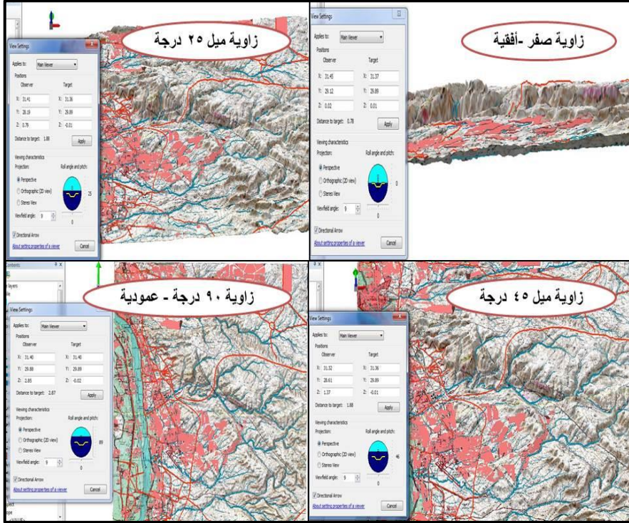
المصدر: من الباحث الطالب اعتماداً على برنامج Arc Sene10.5 شكل ١٢: زوايا ميل مختلفة لمنطقة الدراسة من إعدادات الكاميرا الافتراضية ببرنامج
