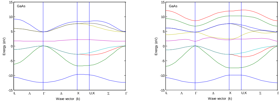
الشكل (5) تركيب حزمة الطاقة لبلورة GaAs نموذج sp^3
