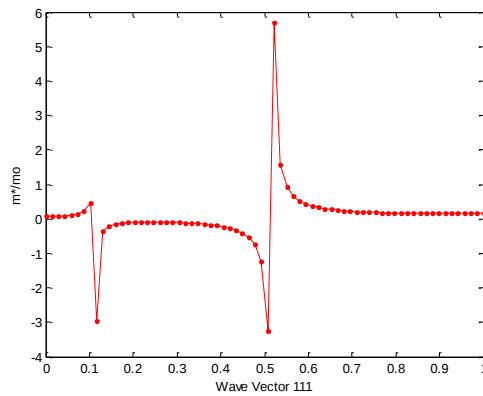
الشكل (7) الكتلة الفعالة m^* لحزمة التوصيل في الاتجاه [111] لبلورة GaAs نموذج sp^3s^* باستخدام طريقة الربط المحكم الشكل (8) الكتلة الفعالة m^* لحزمة التوصيل في الاتجاه [111] لبلورة GaAs نموذج sp^3 باستخدام طريقة الربط المحكم
