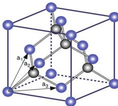
الشكل (1) وحدة الخلية لترتيب بلورة كبريتيد الزنك
