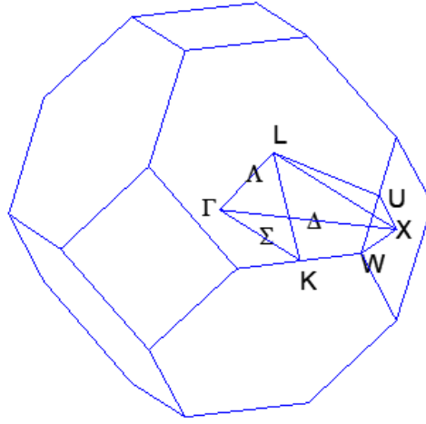
الشكل (2) منطقة برليون الأولى لشبكة بلورية مكعبة ممركة الوجه FCC مع بعض نقاط التناظر العالي
