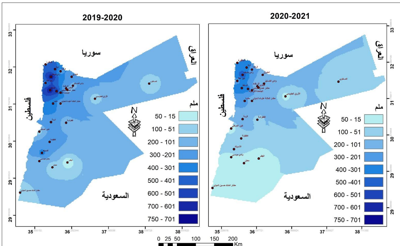
شكل (1): اجمالي الهطول المطري (مم) للأردن (2019-2021).
