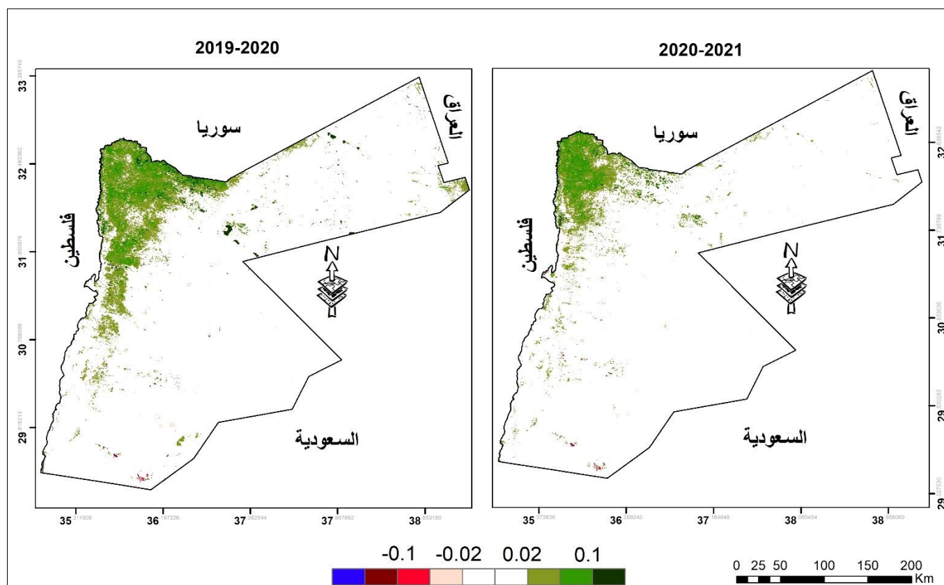
شكل (4): الانحراف عن المعدل للأردن (2021-2019).
