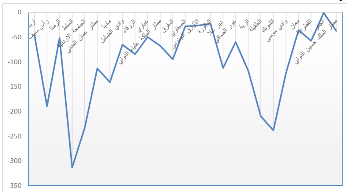
شكل (2): تراجع الاداء المطري للأردن للموسم (2021-2020) عن الموسم (2020-2019) على مستوى المحطات. المصدر: عمل الباحثة بالاعتماد بيانات دائرة الارصاد الجوية، 2021.
