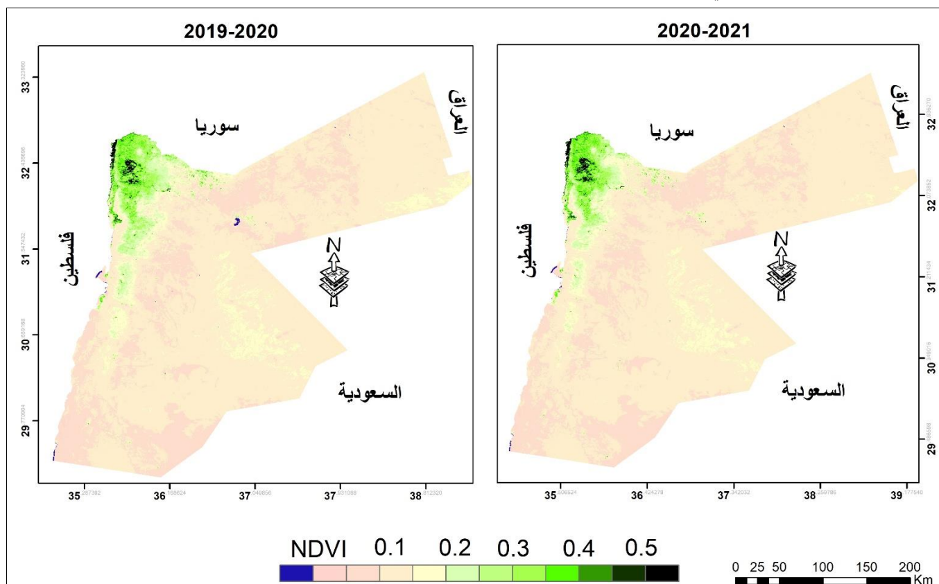
شكل (3): معدل مؤشر الاختلاف النباتي المعايير NDVI للأردن (2021-2019).
