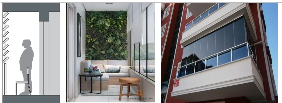
شكل رقم (١٢) استخدام الزجاج للتحكم في المناخ الداخلي للشرفة (١١) .
