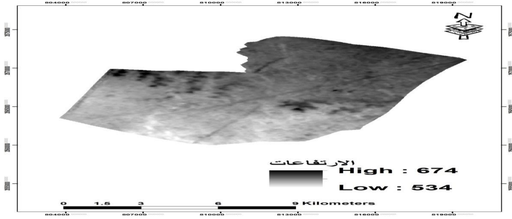
الشكل 2: توزيع قيم الارتفاعات (نموذج الارتفاعات الرقمي (DEM))
