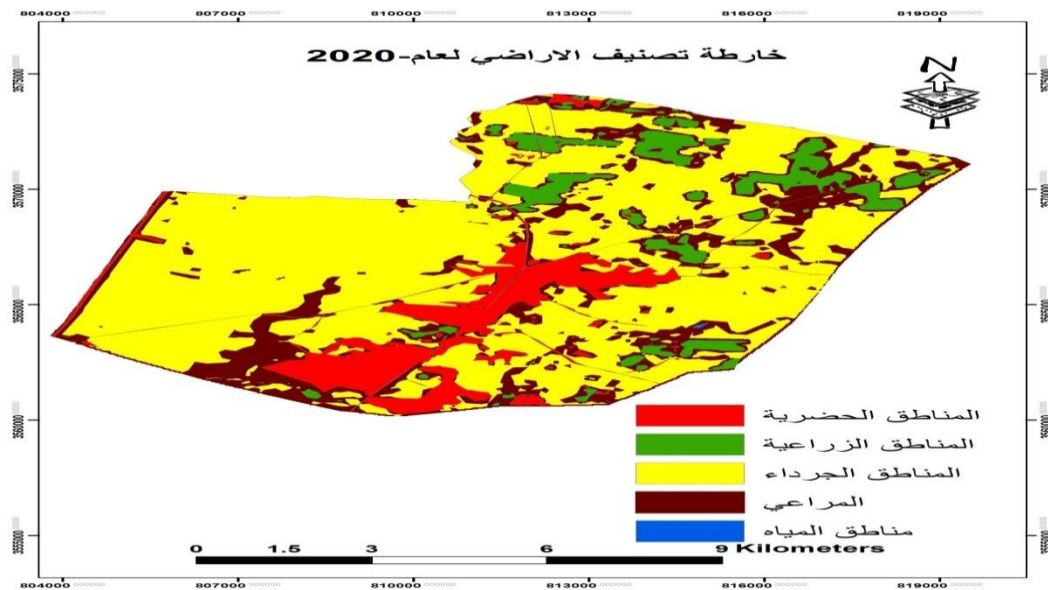
الشكل 6: أنواع الغطاء الأرضي للمرئية الفضائية لعام 2020
