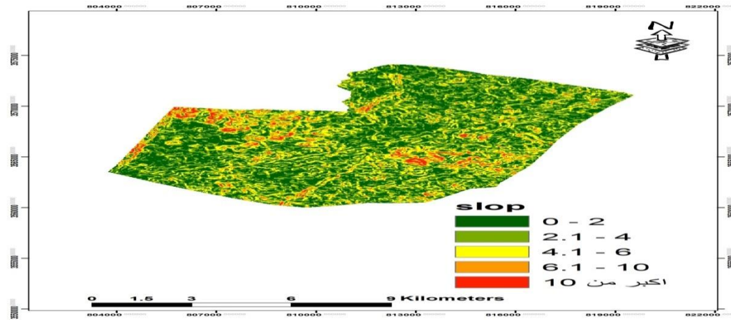
الشكل 3: خارطة درجات الانحدار التي تم اشتقاقها من نموذج الارتفاعات الرقمية (DEM) لمنطقة الدراسة
