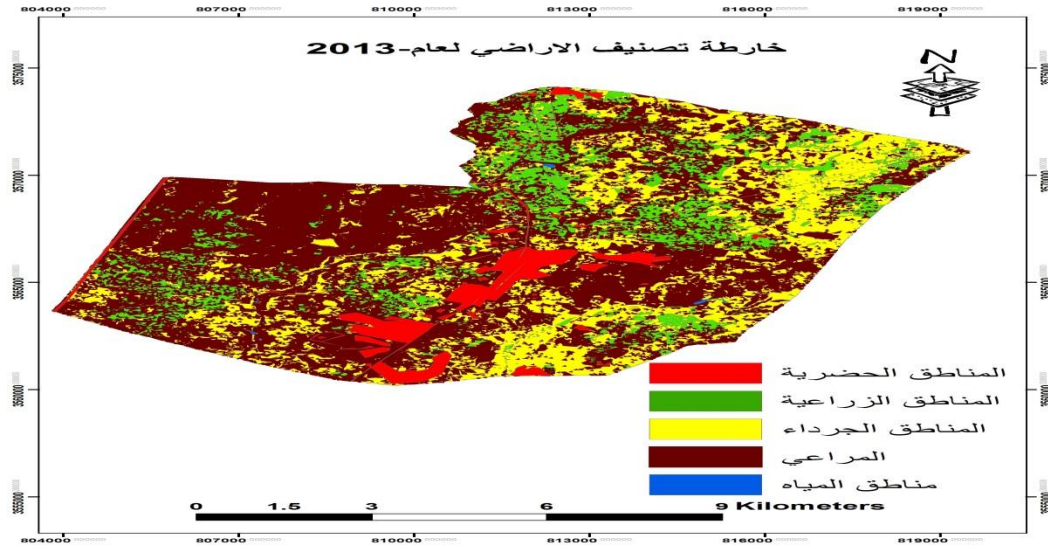
الشكل 5: أنواع الغطاء الأرضي للمرئية الفضائية لعام 2013
