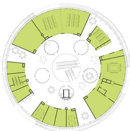
شكل (٦) المسقط الأفقي للدور الأول.
