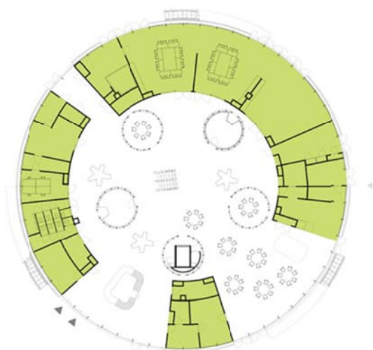
شكل (٥) المسقط الأفقي للدور الأرضي.
