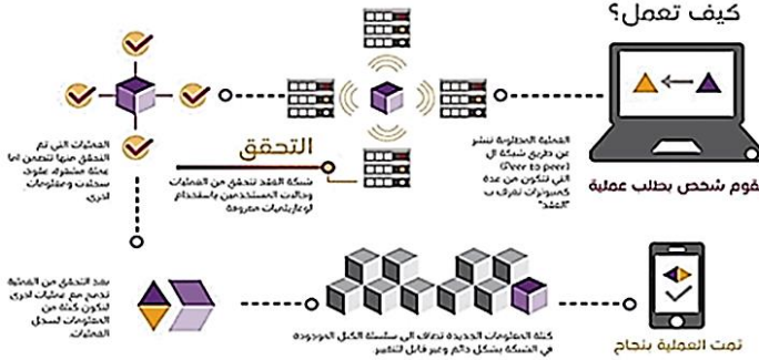
الشكل رقم (03): آلية عمل تقنية البلوك تشين
