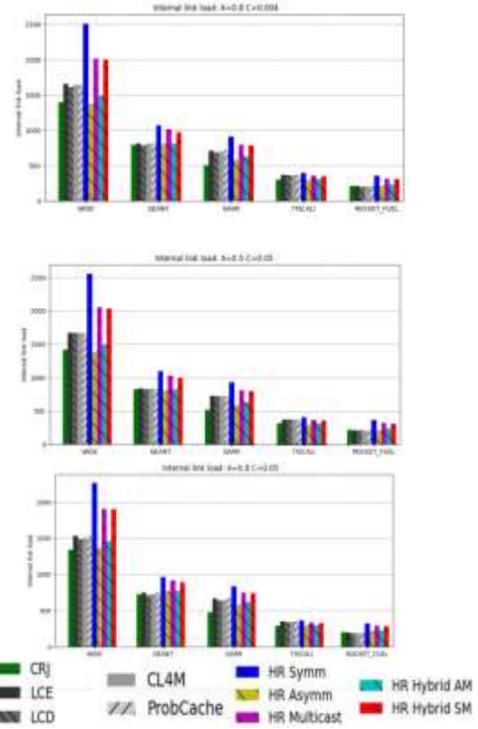
الشكل (8) مقارنة معدلات الحمل على المسار C=0.004 ، C=0.05
