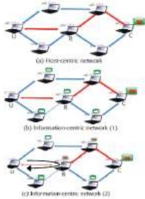
الشكل (1) مقارنة بين الشبكات المتمحورة حول المضيف والمتمحورة حول المعلومات
