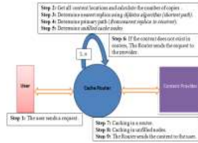
الشكل (2) مخطط عمل خوارزمية CRJ
