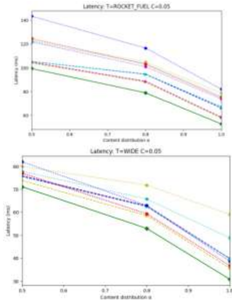
الشكل (7) مقارنة معدلات التأخير C=0.05
