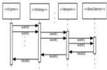
الشكل(4) مخطط ال Sequence Diagram لتنفيذ التجربة في Icarus
