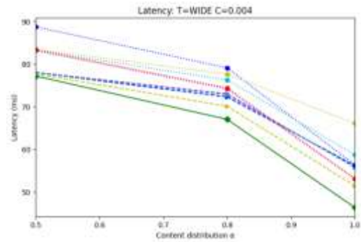
الشكل (6) مقارنة معدلات التأخير C=0.004
