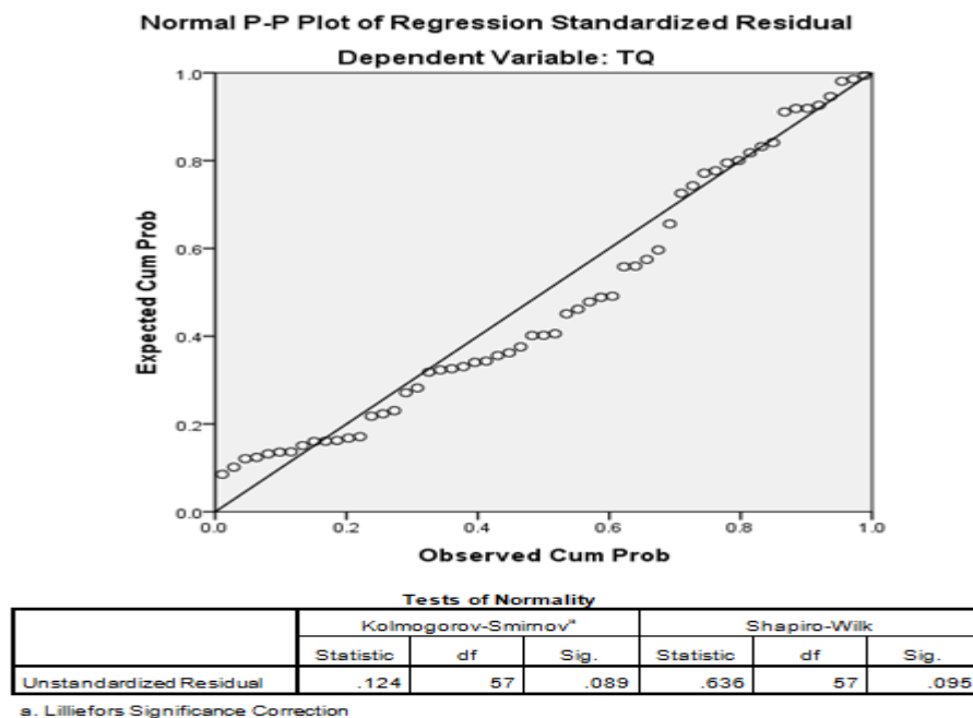
الشكل رقم (4-1): التوزيع الطبيعي للبواقي في نموذج الدراسة الأول
