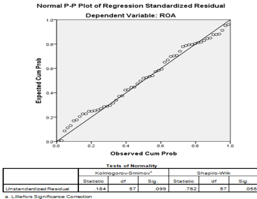
الشكل رقم (4-2): التوزيع الطبيعي للبواقي في نموذج الدراسة الثاني
