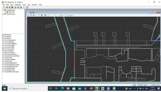
شكل (6) يوضح التحليل البصري لصالات الأنتظار لمطار أسطنبول الدولي
