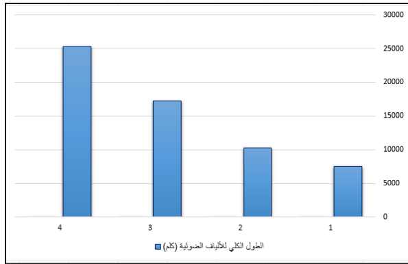
شكل (8): الطول الكلي للألياف الضوئية بالكيلومتر مقابل عدد الوصلات بين المدن
