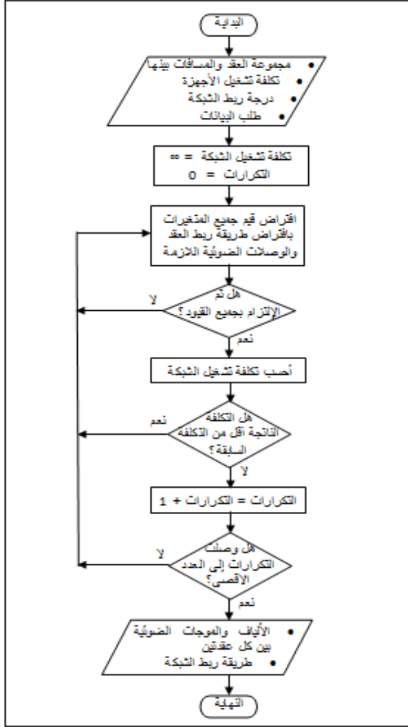
شكل (2) مخطط خطوات نموذج ربط مدن الشبكة
