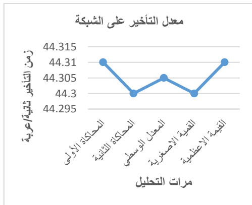
الشكل (6) معدل التأخير على شبكة شوارع مدينة دمشق
