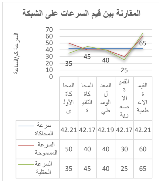
الشكل (8) مقارنة السرعة الوسطية الحقلية والمسموحة
