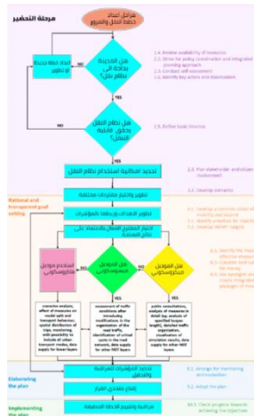
الشكل (3) مراحل معالجة خطط النقل والمرور. (P. L. Schiller, and other, 2011)
