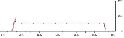
الشكل (12) تدفق الحزم في طوبولوجيا fat-tree بعد تطبيق الآلية
