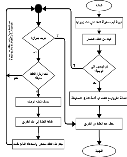
الشكل (5) مخطط تدفق إجرائية حساب كافة المسارات بين المصدر والوجهة
