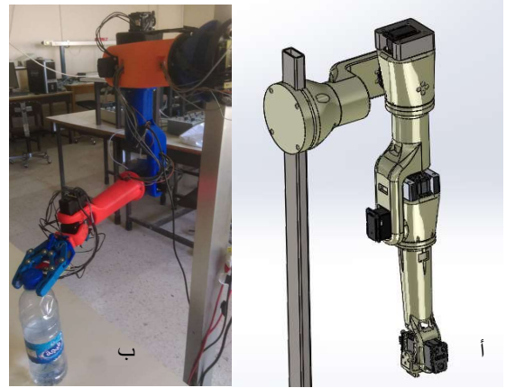
الشكل 9 أ. التصميم النهائي للذراع المخبرية ذات سبع درجات حرية رابطية ب. الذراع الزويوتية المخبرية المنفذة.
