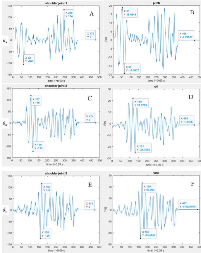
الشكل 11 خطأ ملاحقة اتجاه محدد أثناء تحريك روابط مفصل الكتف يدويًا بسرعات زاوية لا تتجاوز 140^\circ/s . يقابل كل دوران في الفضاء العمليتي (pitch roll yaw) دوران في الفضاء الزائدي \theta_1, \theta_2, \theta_3 على الترتيب (الشكل (ACF))، حيث تم إجراء الاختبار بتحريك روابط مفصل الكتف بشكل متسلسل ثم بشكل مركب لمعرفة الخطأ السكوني المبين في الأشكال BDF.
