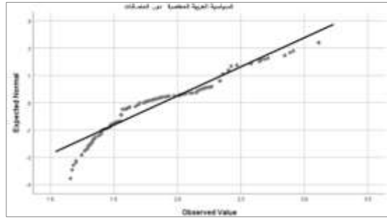
الشكل (94): رسم بياني لخطية المصنفات السياسية العربية المعاصرة
