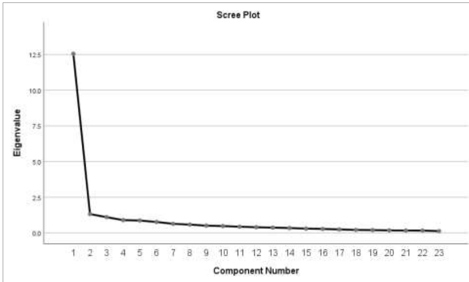
الشكل (96): التمثيل البياني لقيم الجذور الكامنة للعوامل المكونة للأداة
