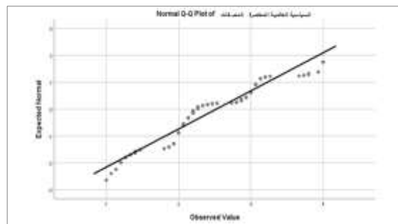
الشكل (95): رسم بياني لخطية المصنفات السياسية العالمية المعاصرة
