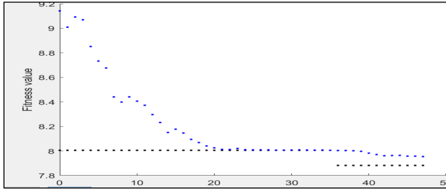
شكل (4) : افضل دالة لياقة عند (M=55150)
